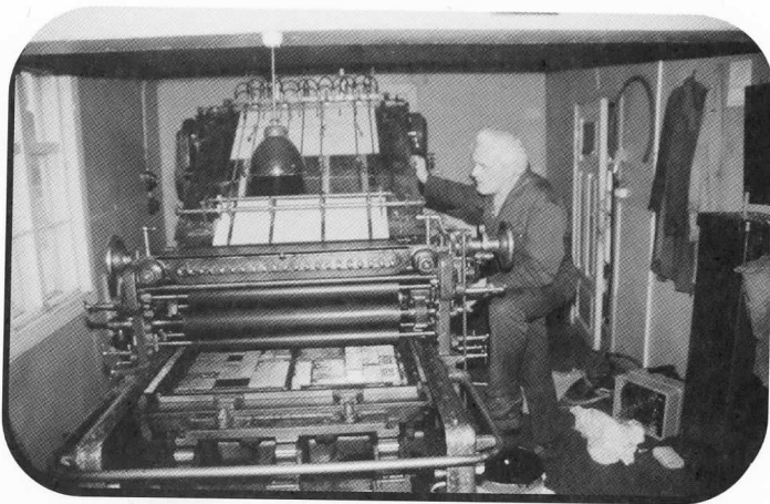
Torbjørn med Nibiola trykkpressen i gang.
